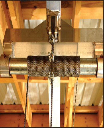
Cable Rollers
